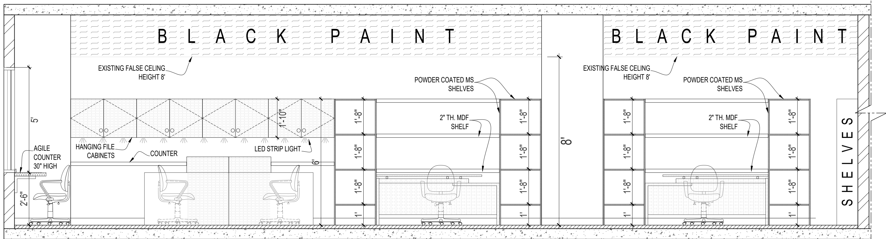
ELEVATION B SCALE: 3/8" = 1'-0"
