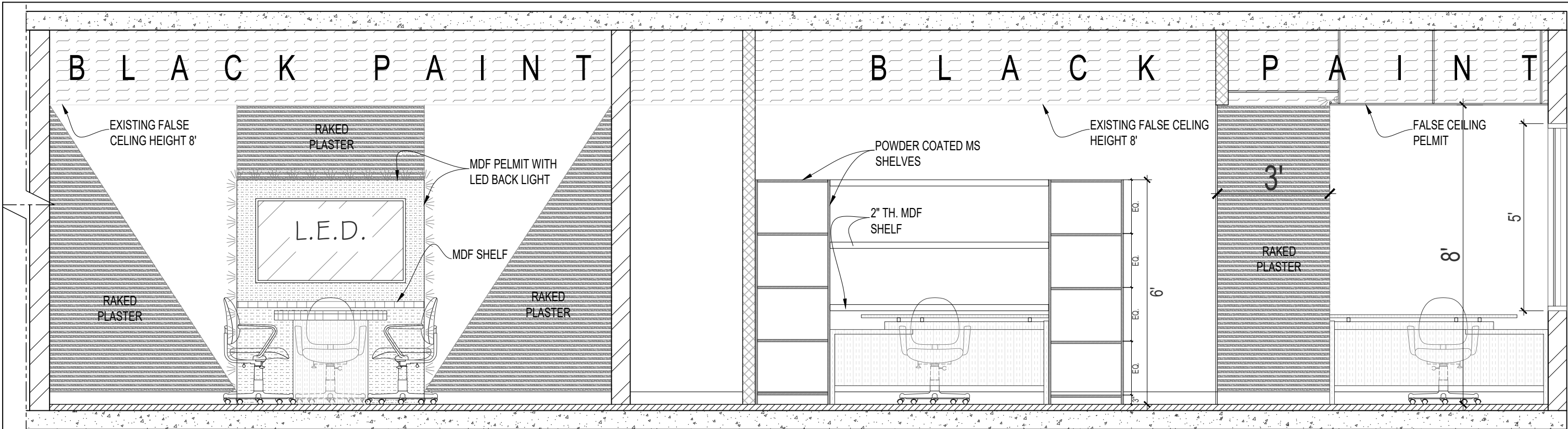
ELEVATION A SCALE: 3/8" = 1'-0"
