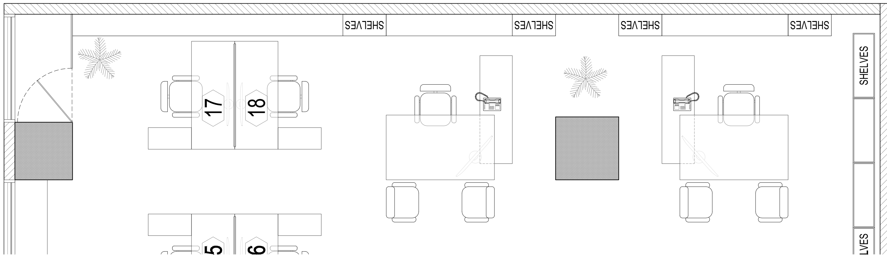
PART PLAN SCALE: 3/8" = 1'-0"
